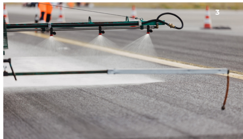
1 Onyxauftrag | 2 digitale Einstellung der Auftragsmenge | 3 eshabit Onyx Primer als Haftgrund
